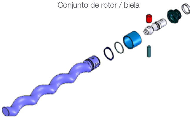
Conjunto de rotor / biela
